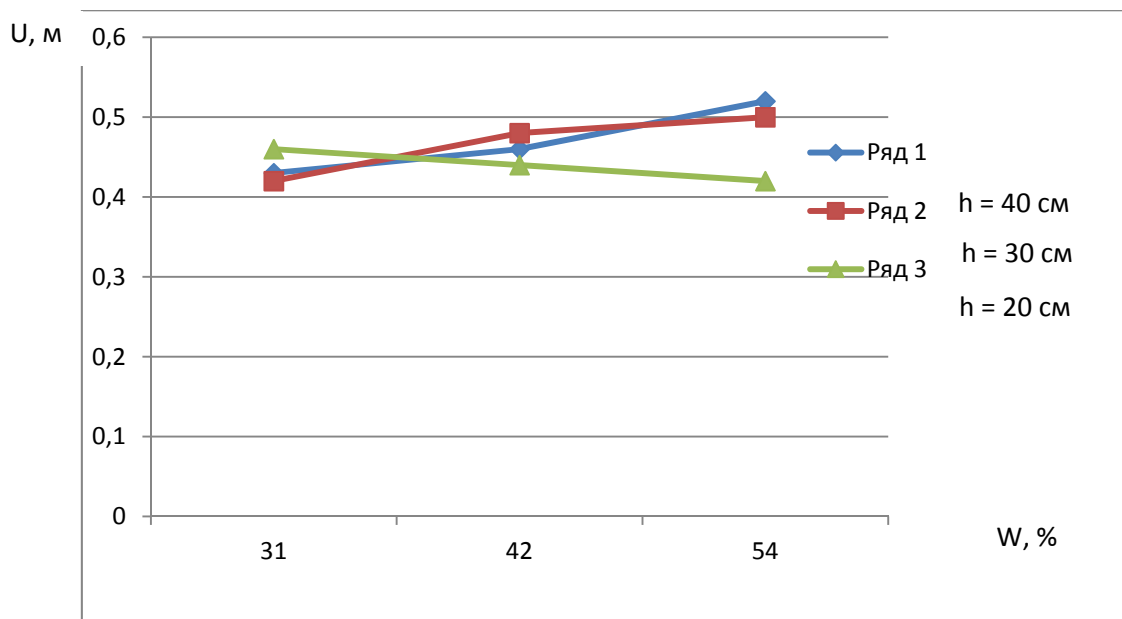
Рис. 5. Залежність показів ПВГТ від вологості ґрунту Fig.5. Dependence of the DDDS indications on soil moisture
