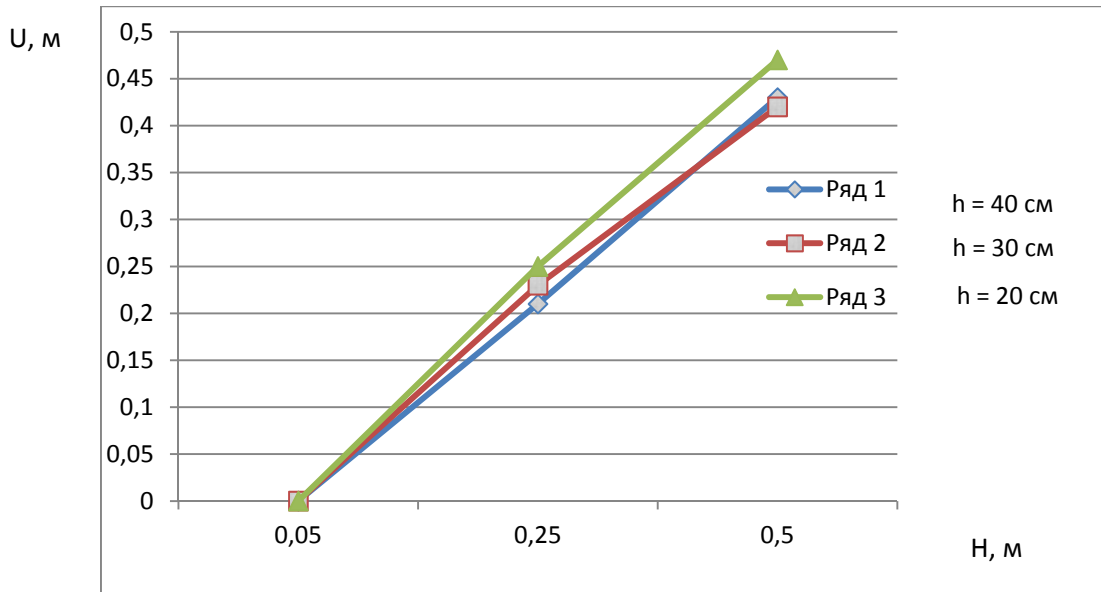
Рис. 4. Залежність показів ПВГТ від глибини залягання ущільненого шару ґрунту Fig.4. Dependence of the DDDS indications on the depth of the compacted layer of soil
